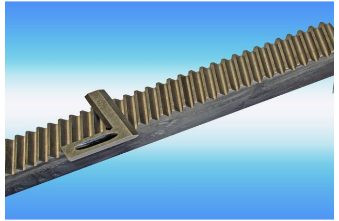
Schrägverzahnte Zahnstangen
